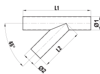
Abzweig 45°
