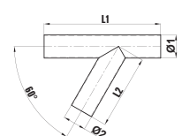
Abzweig 60°
